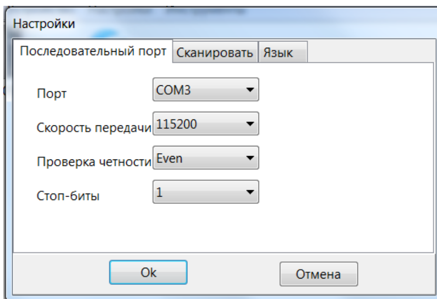
Настройка последовательного порта
